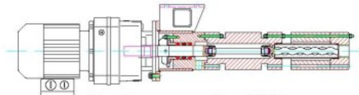
Dosierpumpe Typ MPS mit Sonderwelle
