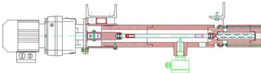
Stopfbuchslose Dosierpumpe Typ MPos mit Zulaufüberwachung
